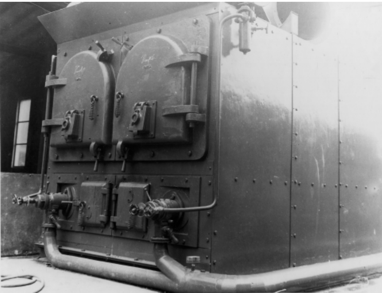
15 Transportabel, oliefyret dobbelt-muffelovn til kz-lejre af Topf & Söhne, 1940
